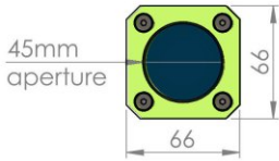
Front Lid
